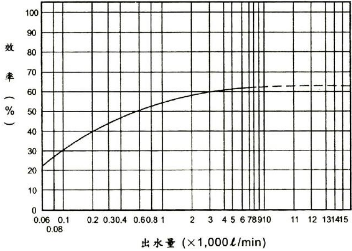
附圖3 幫浦效率曲線
