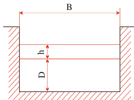
圖 12 全幅堰
