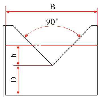
圖 10 直角三角堰
